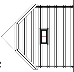
Zijgevel Links
