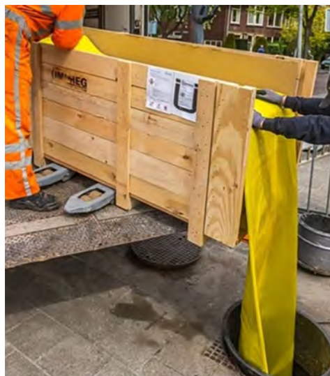
Aanbrengen van de glasvezelkous op het terrein
