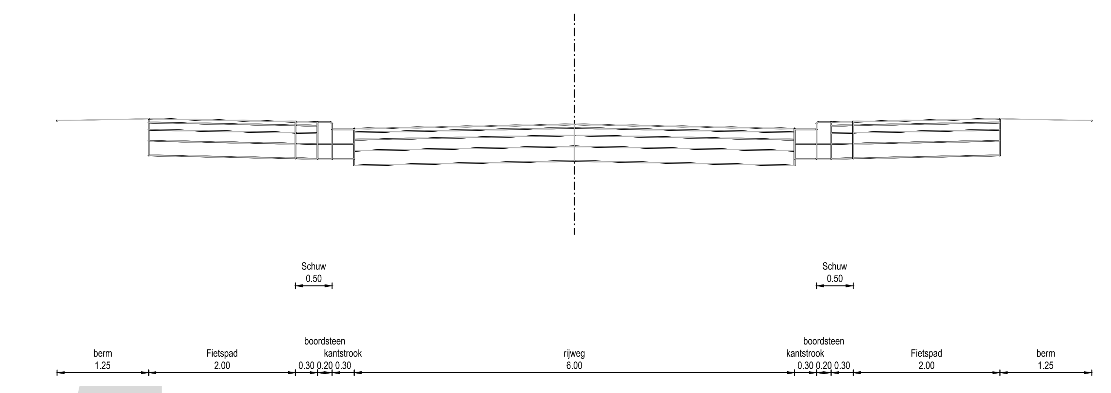
Variant 1 fietspaden 2m aanliggend
